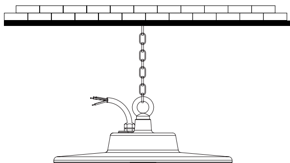
Montaža na lanac-sajlu
